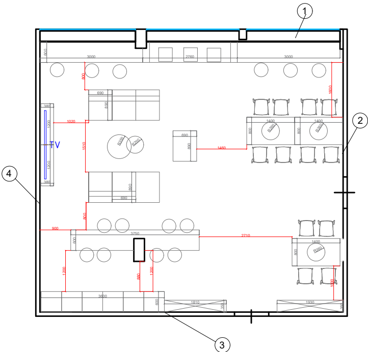
Baldų planas ir matmenys, sienų išsklotinės
