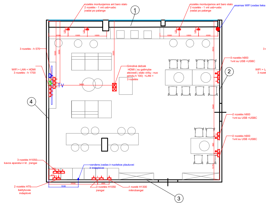
Kištukinių lizdų planas
