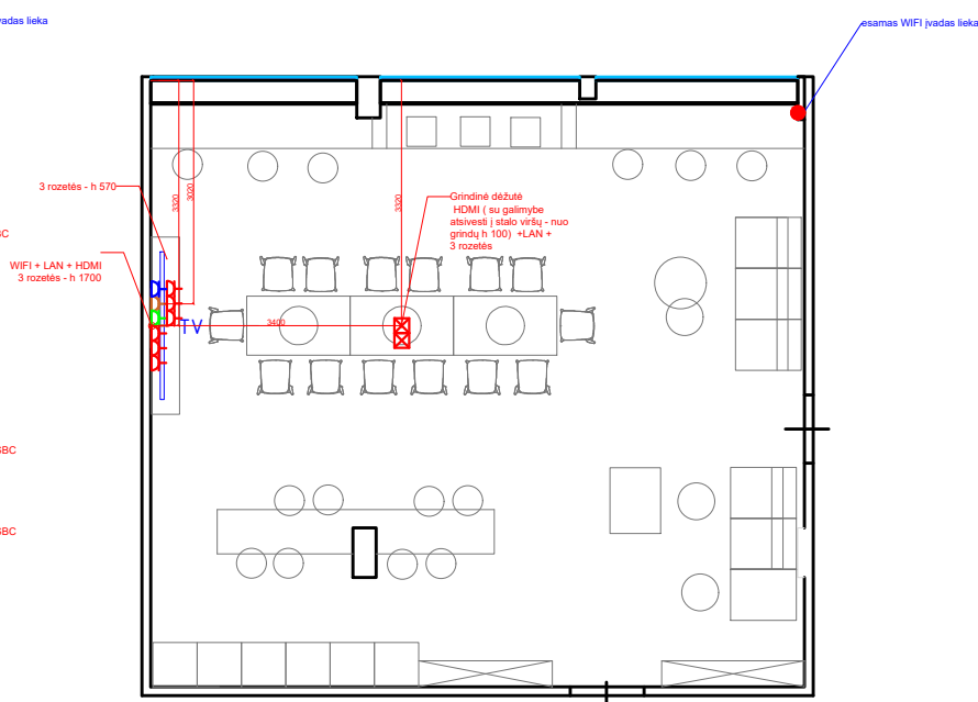
Kištukinių lizdų planas posėdžių erdvei
