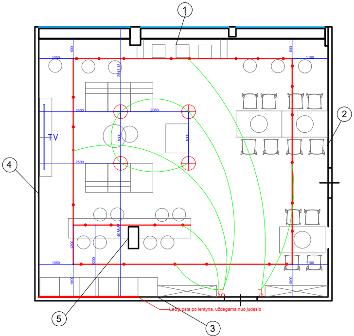
Apšvietimo planas ir jungikliai
